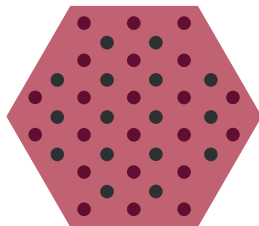
Vulkanischer Porphyry
